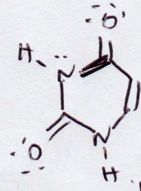
uracil
