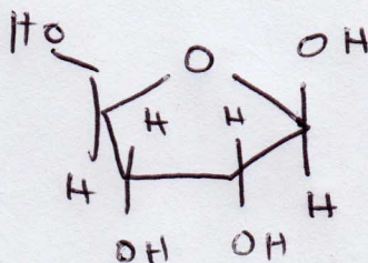
ribose
