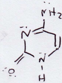
cytosine
